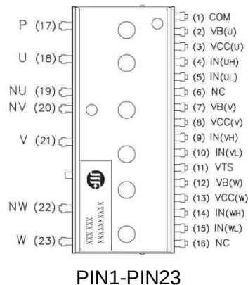
PIN1-PIN23
