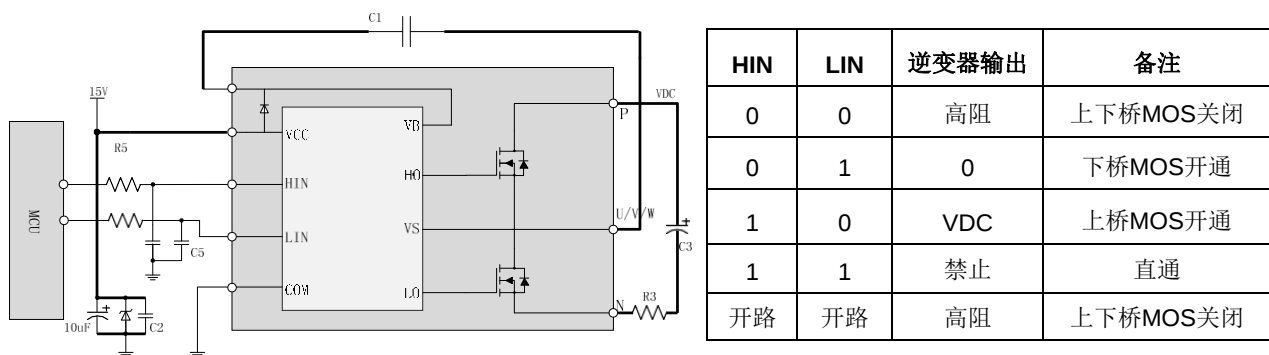
图 9: MCU 接口和自举推荐电路
