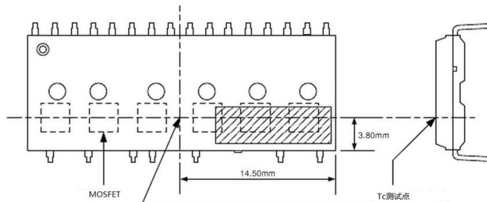
图 5: 壳温 T_c 测试点
