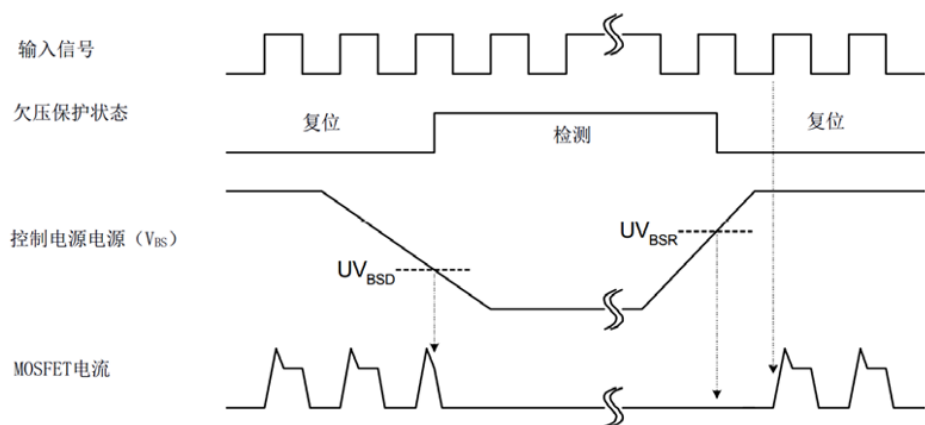
图 8: 欠压保护时序图(高侧)
