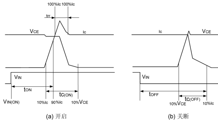
图 4: 开关时间定义
