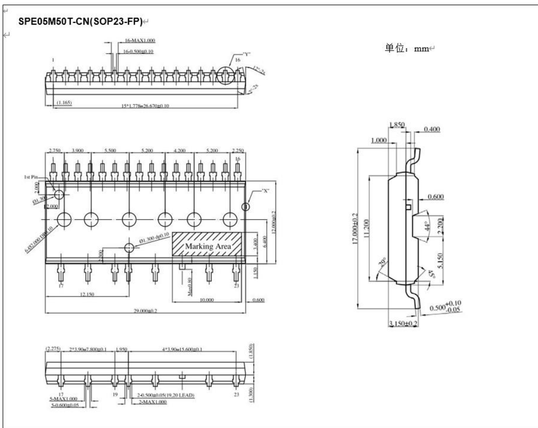
图 12: SPE05M50T-CN 封装外形图
