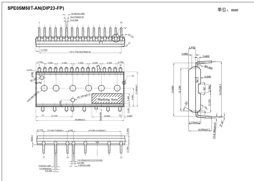
图 11: SPE05M50T-AN 封装外形图
