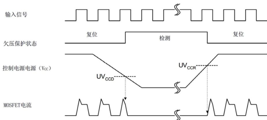
图 7: 欠压保护时序图(低侧)
